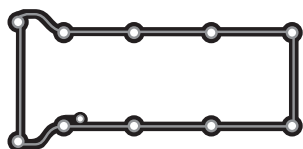
JVS-303-43 - XS6E6584AB/6710A2B Junta Tapa Válvula Superior Junta Tampa Válvula Superior
