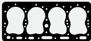
TC-301-05 - 2009064/2000047 Junta Culata de Cilindros Junta Cabeçote
