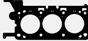
TC-636-11 4921510/6F9E6083AB/AJ0310272 Junta Culata de Cilindros (Izquierda) Junta Cabeçote (Esquerda)
