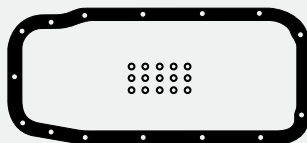
JC-306-30 - 90572656 90409693/93335433 Junta Cártier c/ arandelas limitadoras de apriete Junta Carter c/ aruelas limitadoras de ajuste
