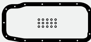
JC-306-30 - 90572656 90409693/93335433 Junta Cártel c/arandelas limitadoras de apriete Junta Carter c/arruelas limitadoras de ajuste
