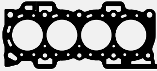
TC-124-15 - 1111587105/06 Junta Culata de Cilindros Junta Cabeçote
