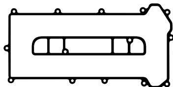
JVS-349-43 - 1S7G6584AE/LF0110230 Junta Tapa Válvula Superior Junta Tampa Válvula Superior
