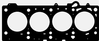
TC-664-11 - 4884407AA/48844443AD Junta Culata de Cilindros Junta Cabeçote
