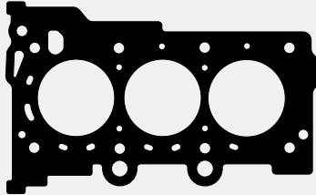
TC-651-11 Junta Culata de Cilindros Junta Cabeçote
