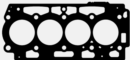
TC-895-11 - 9676157680/0209JF/JN Junta Culata de Cilindros Junta Cabeçote
