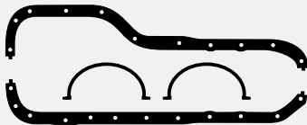
JC-290-30 Junta Cártér Junta Carter
