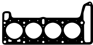
TC-542-15 - 21011003020 Junta Culata de Cilindros Junta Cabeçote
