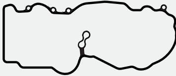
Junta Tapa Válvulas Junta Tampa Válvulas
