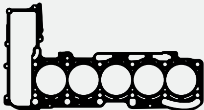
TC-953-07 - 07K103383F Junta Culata de Cilindros Junta Cabeçote
