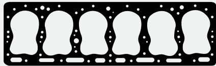
TC-199-05 - 19915/733567 Junta Culata de Cilindros Junta Cabeçote
