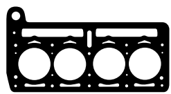
TC-208 - 4064640 Junta Culata de Cilindros Junta Cabeçote
